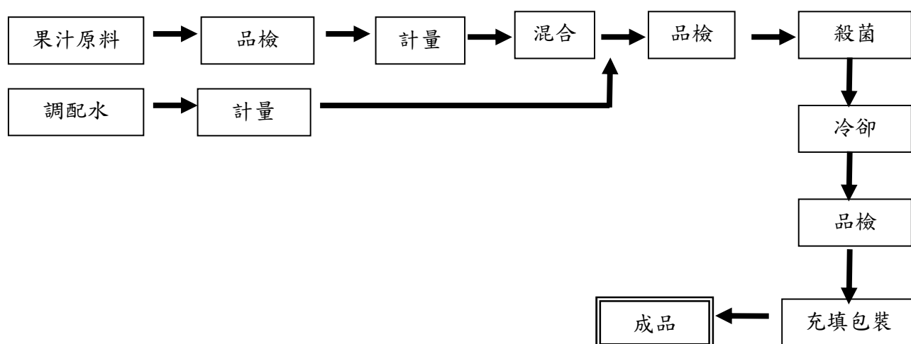
(3)果汁製造流程圖
