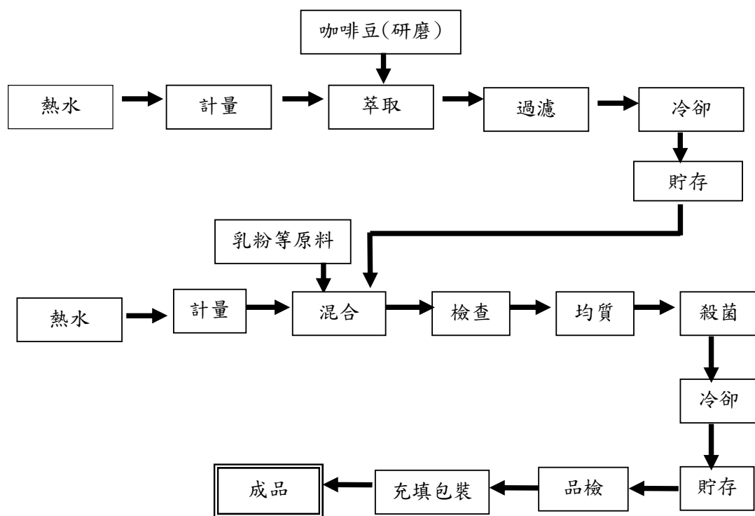
(4)咖啡製造流程圖
