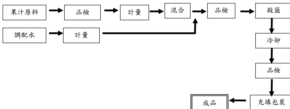
(3)果汁製造流程圖
